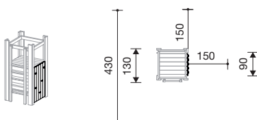
3.68305 hellende evenwichtsbalk voor hut H 1,50 m
