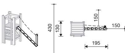
3.69433 klimkoord voor hut H 1,00 m
