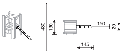
3.69430 klimkoord voor hut H 1,50 m
