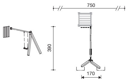
3.19802 enkele aanbouschommel met stalen dwarsbalk
