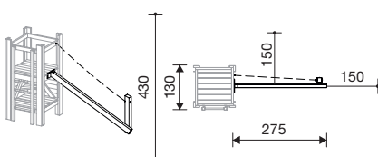
3.69515 klimstam met kettingleuning voor hut H 1,50 m
