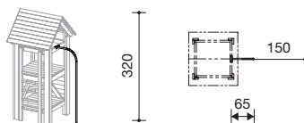
3.69480 gebogen glijstang voor hut H 1,50 m
