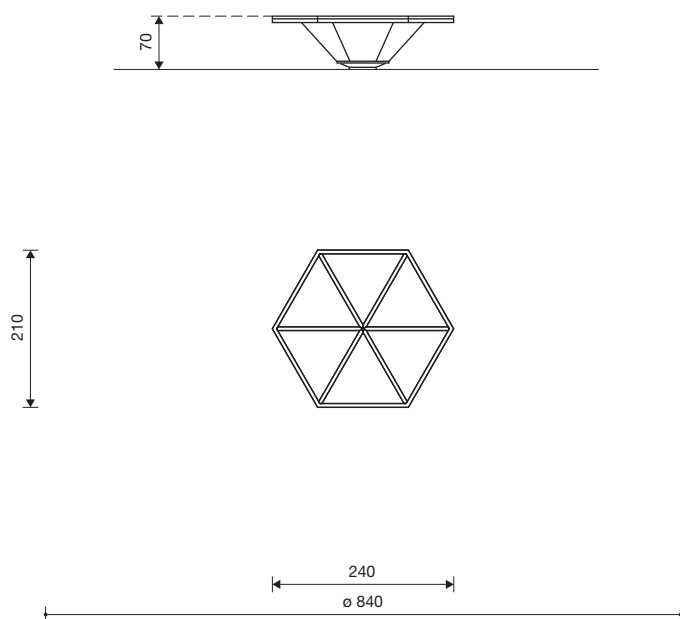
10.73300 grote balanceerschijf ø 3,40 m
