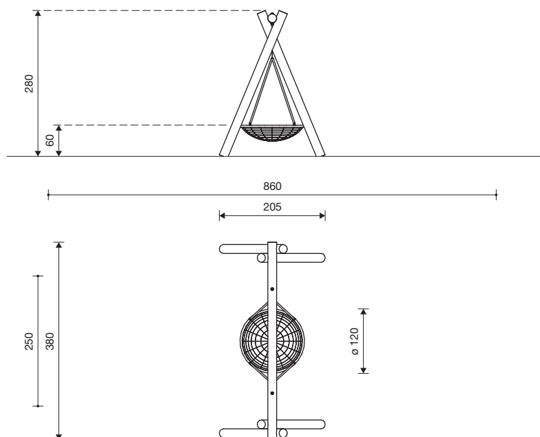
6.14500 vogelnestschommel
