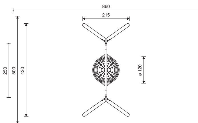
6.14520 vogelnestschommel met stalen dwarsbalk
