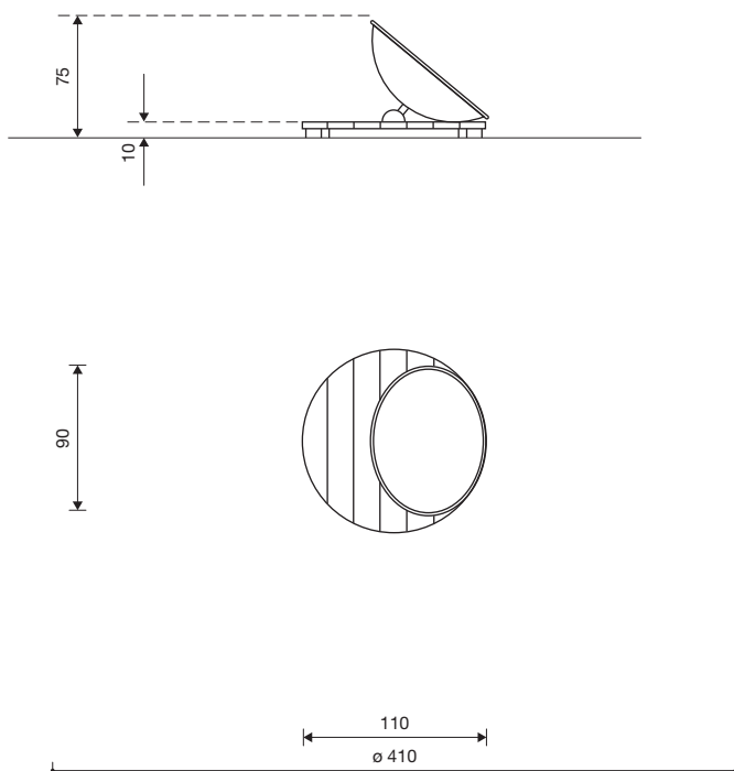
6.27300 wiebelkuip
