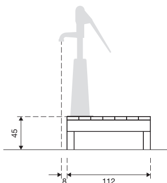
5.19000 pompplatform
